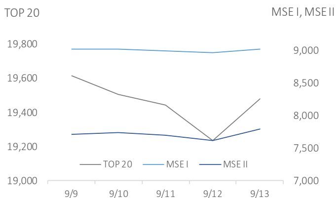
MSE Индекс
